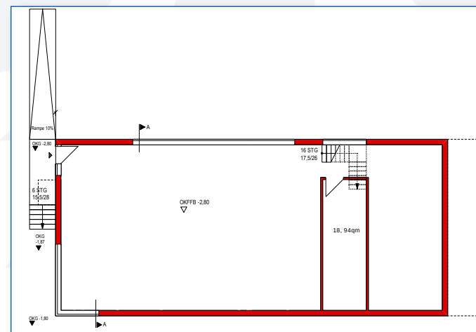
Untergeschoss
